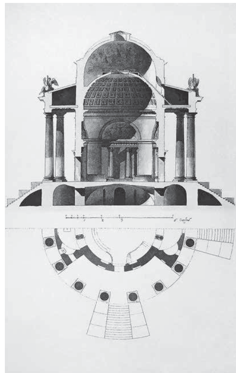
Воскресенская (Никольская) церковь-мавзолей. Разрез и часть плана. Проект
