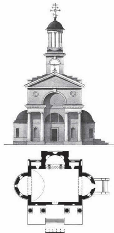
Владимирская (Никольская) церковь в селе Горницы. Фасад и план. Обмерный чертёж
