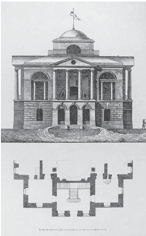
Дом В. С. Томары на окраине Петербурга. Проект
