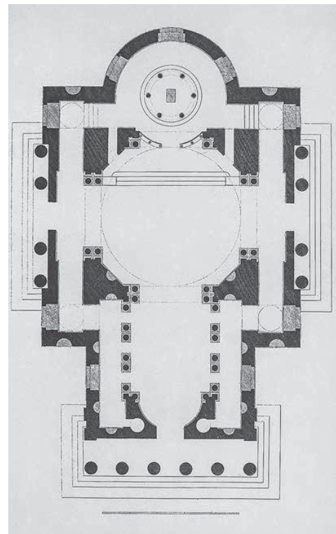
Собор Св. Иосифа в Могилёве. План. Проект
