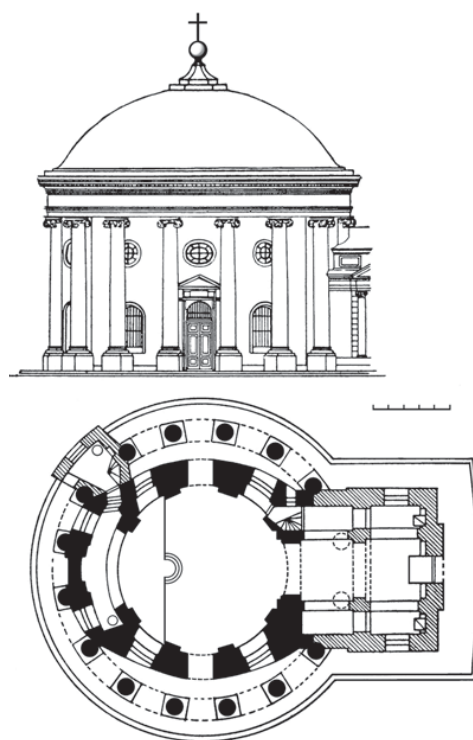
Церковь Троицы «Кулич и Пасха». Фасад и план
