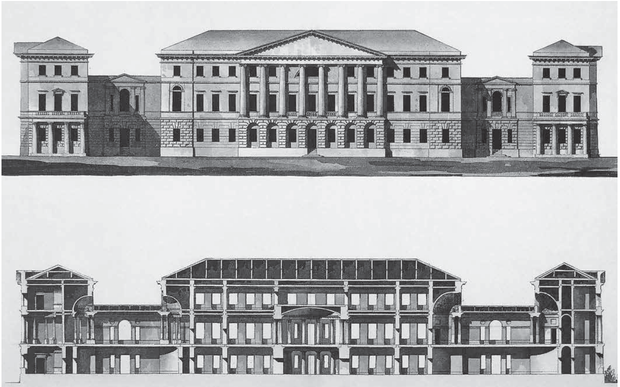
Загородный дом А. И. Воронцова в усадьбе Вороново под Подольском. Проект
