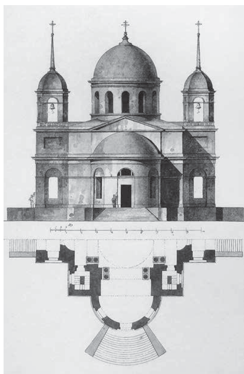
Троицкая церковь в усадьбе Дохновичи Черниговской губернии. Проект
