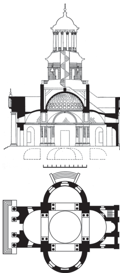
Церковь Св. Екатерины. Разрез и план
