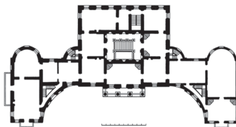
Дом в усадьбе Никольское-Черенчицы. План
