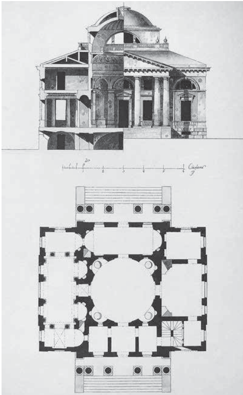
Дом П. А. Соимонова на Выборгской стороне в Петербурге. Проект
