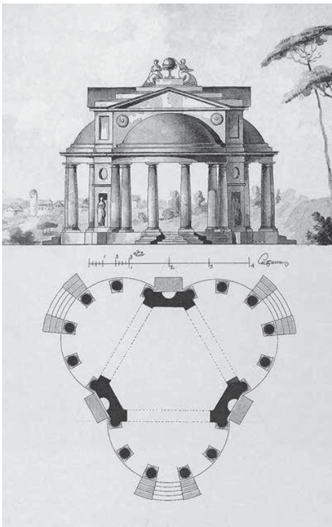
Павильон с тремя экседрами в усадьбе Знаменское-Раёк. Проект
