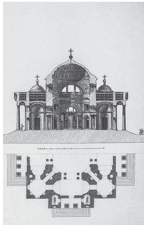
Собор Борисоглебского монастыря. Разрез и часть плана. Проект
