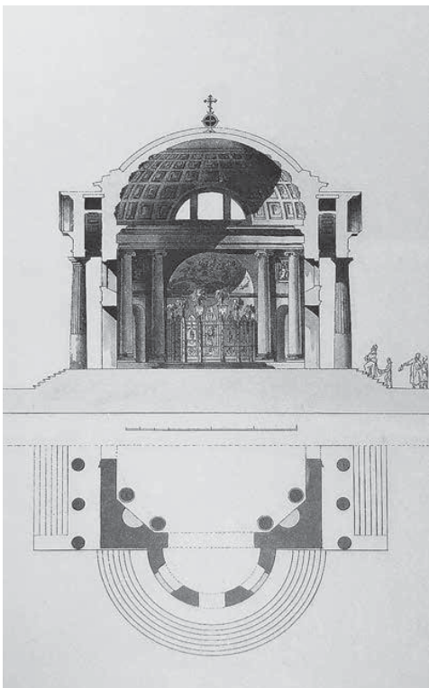
Казанская церковь в селе Арпачёво. Разрез и часть плана. Проект
