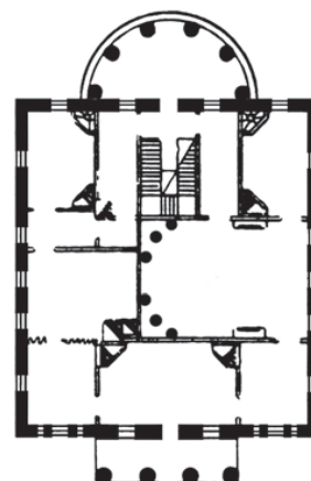
Дом Г. Р. Державина в усадьбе Званка Новгородской губернии. Обмерный чертеж
